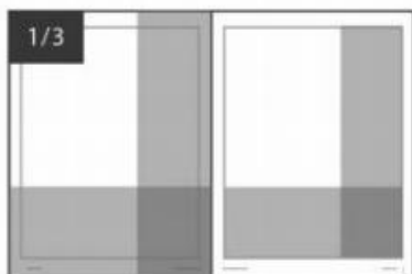
HORIZ 210x92 mm INNER 190x75 mm VERT 69x276 mm INNER 60x246 mm
